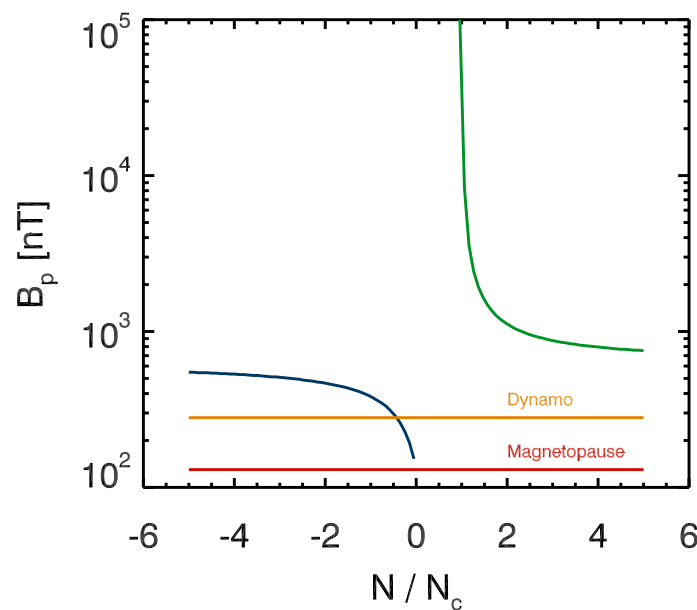
Abbildung 6.2: Planetares Dipolfeld in Abhängigkeit der normierten Dynamozaahl. Die blaue Kurve markiert den Lösungsast mit einem schwachen Oberflächenfeld, während die grüne Kurve die Lösungen mit einem starken Feld anzeigt. Die rote Linie zeigt die minimale Feldstärke für eine Magnetopause oberhalb der Planetenoberfläche an. Die orangefarbene Linie markiert den Übergang von Magnetokonvektion hin zu einem echten Dynamoprozess. Abbildung nach Glassmeier et al. (2007).
