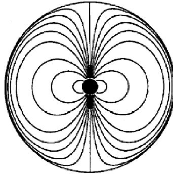
Abbildung 3.8: Kompensation eines Dipols durch einen Schichtstrom. Die Situation ist hier für den terrestrischen Fall dargestellt. Die Erde ist durch eine schwarze, ausgefüllte Kreisscheibe repräsentiert, während die Magnetopause durch einen Kreis markiert wird. Die schwarzen Magnetfeldlinien deuten an, dass das Magnetfeld auf die Magnetosphäre begrenzt ist und in Bezug zu ihr nur noch tangentielle Komponenten aufweist. Abbildung aus Willis et al. (2000).
