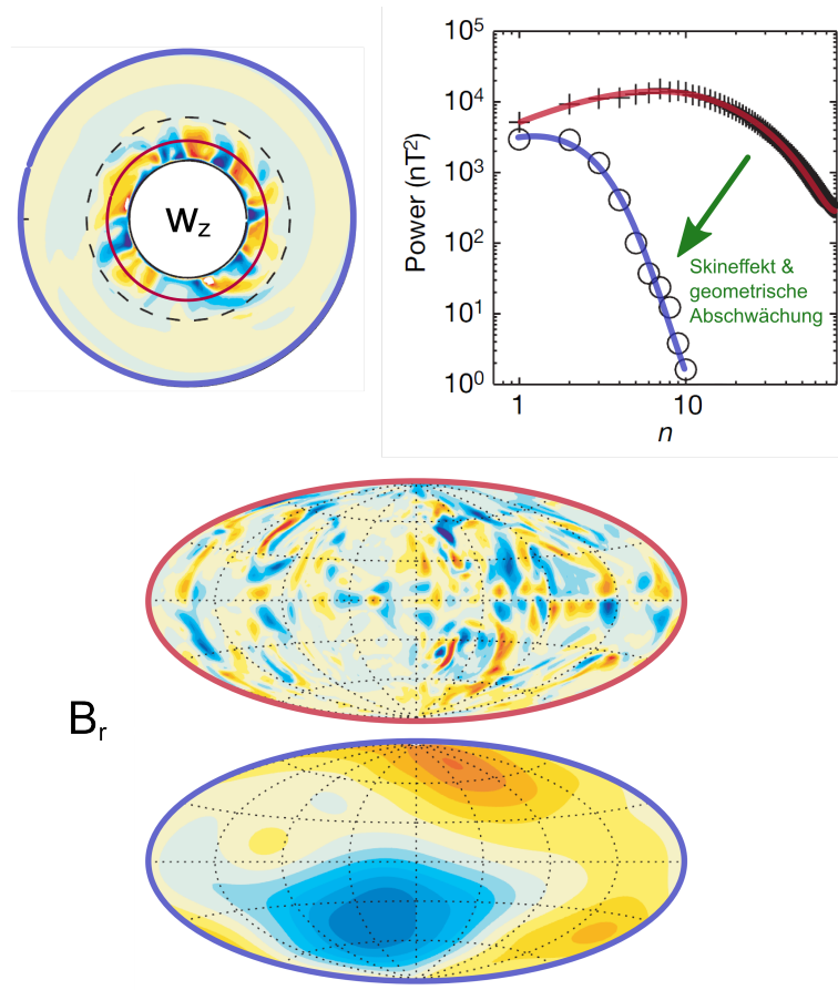
Abbildung 9.7: Dynamomodell für den Merkur nach Christensen (2006). Oben links : Axiale Vortizität. Oben rechts : Magnetische Spektren. Kreuze stehen für das Spektrum im konvektierenden Teil des Kerns und Kreise für das Spektrum an der Oberfläche. Unten : Radiales Magnetfeld. In der oberen Teilabbildung ist das Magnetfeld in der Dynamo-schicht und in der unteren Teilabbildung an der Oberfläche dargestellt. Rot bedeutet hier auswärts und blau einwärts gerichtetes Feld. Einzelabbildungen aus Christensen (2006).
