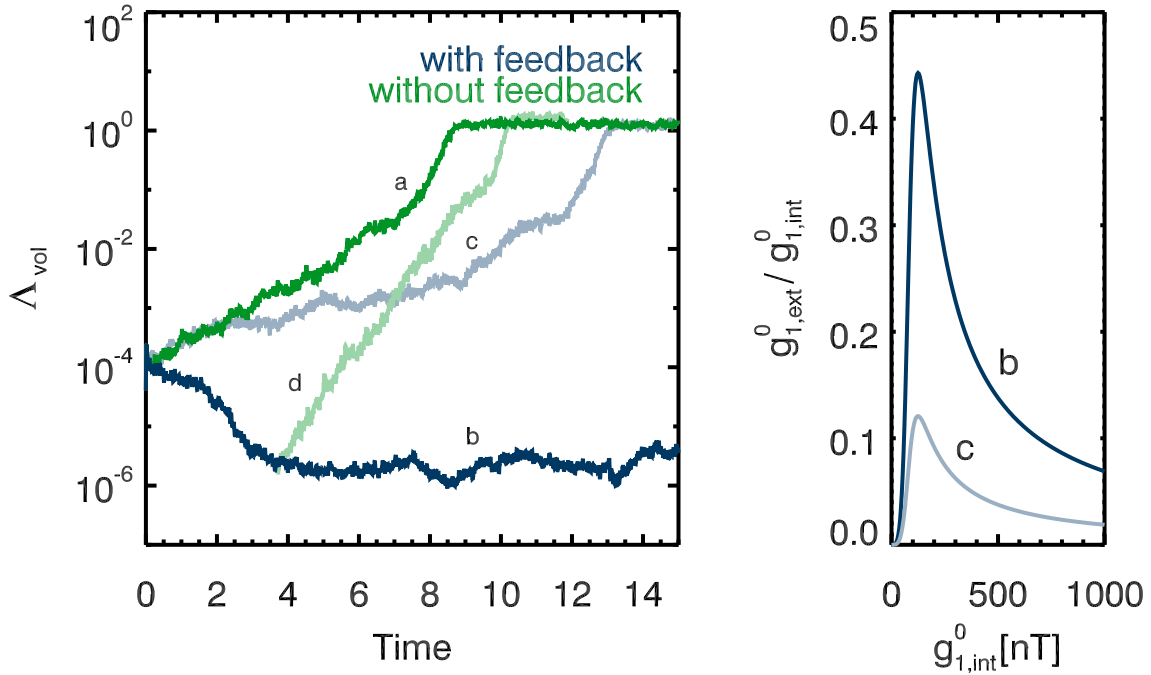
Abbildung 7.5: Links: Volumengemittelte Elsasser-Zahl in Abhängigkeit der Zeit in Diffusionszeiten. Rechts: Relative Antwortfunktion für die links dargestellten Fälle. Fall a: Referenzsimulation ohne Feedback. Fall b: Simulation mit Feedback und relativ starkem externen Feld. Fall c: Simulation mit Feedback und relativ schwachem externen Feld. Fall d: Kontrollsimulation ohne Feedback - ausgehend von der Simulation mit Feedback (b) nach 3 Diffusionszeiten. Abbildung aus Heyner et al. (2011b).
