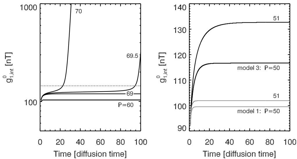
Abbildung 6.7: Links : Zeitliche Entwicklung des internen Dipolfeldes für verschiedene Dynamozahlen für die Antwortfunktion model 2 . Rechts : Vergleich der zeitlichen Entwicklung der Dynamos mit den Dynamo 50 und 51 für die Antwortfunktionen 1 und 3. Abbildung aus Heyner et al. (2010).
